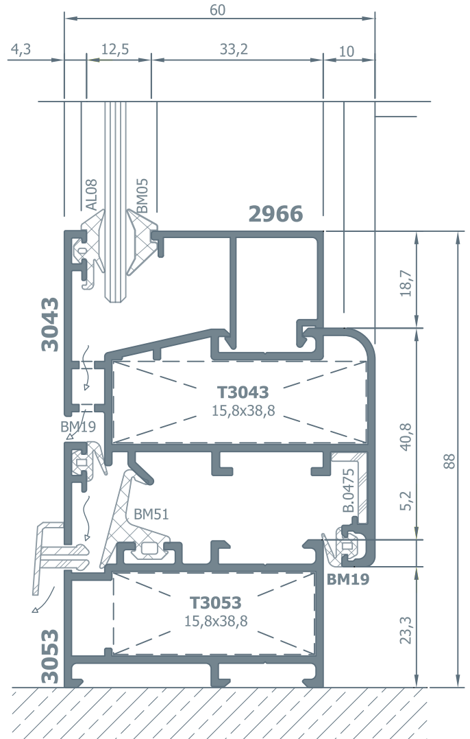
2.2 Detayı Details
