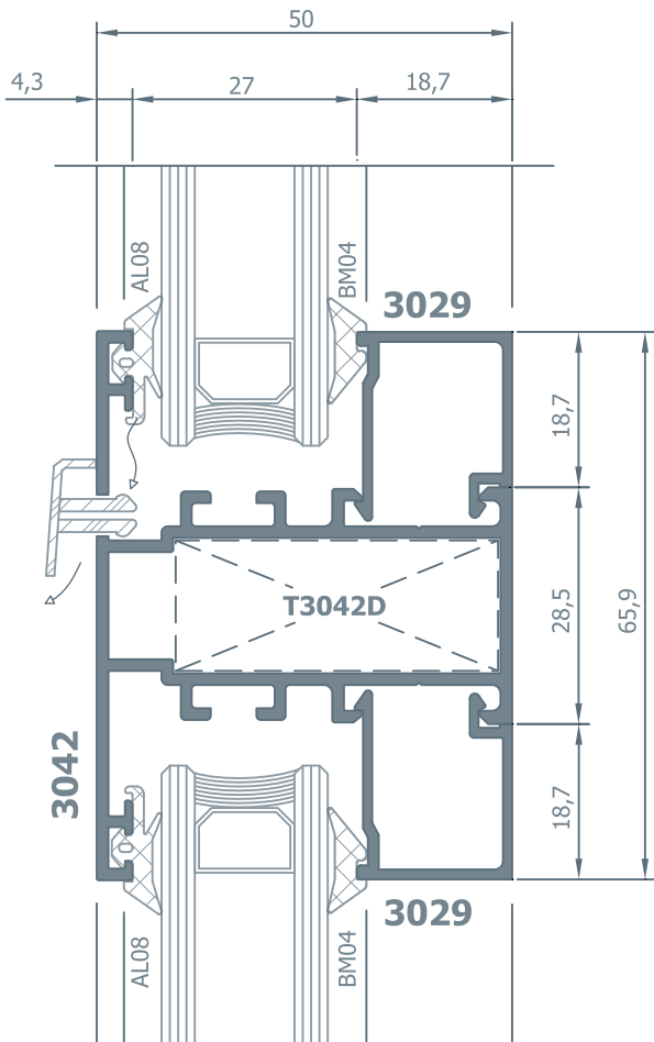
10.10 Detay Details
