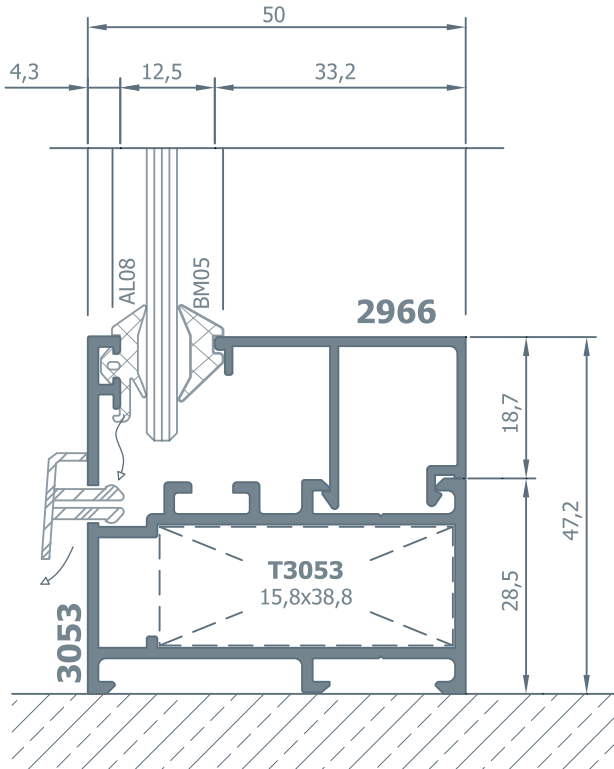
1.1 Detayı Details
