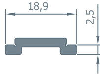
4016 Tij Profili 0.138 kg/m
