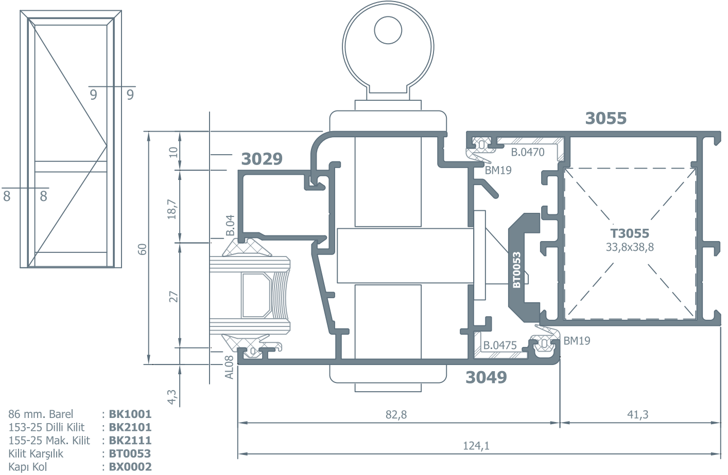
9.9 Detayı Details
