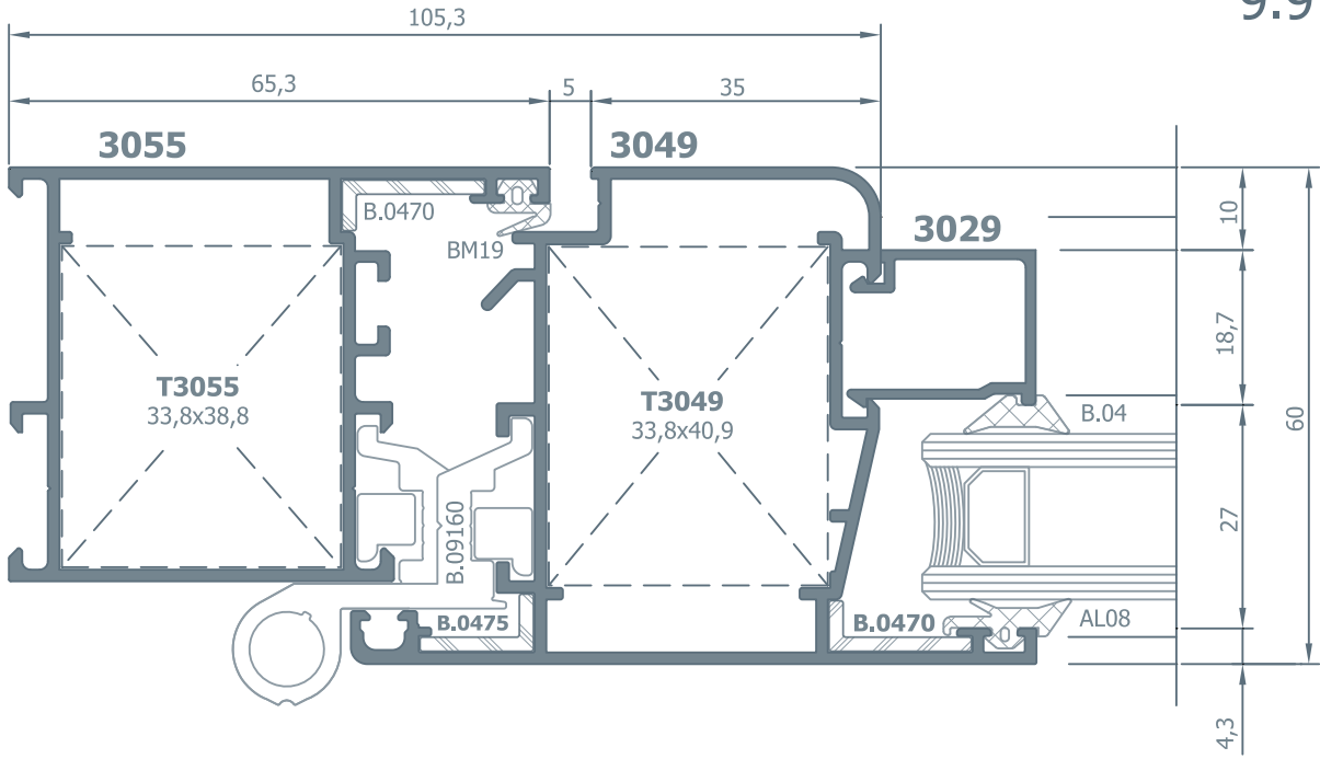
8.8 Detayı Details
