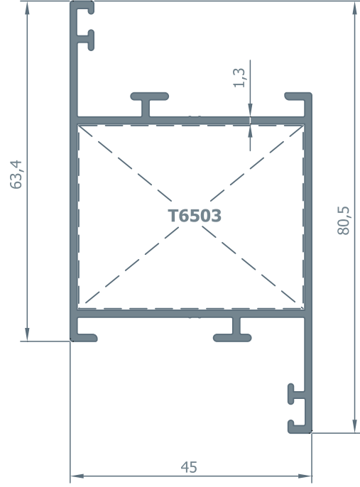
6503 Kanat Profili 0.901 kg/m
