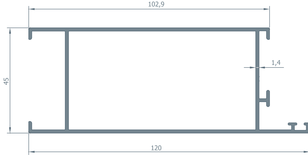
6520 Baza Profili 1.265 kg/m
