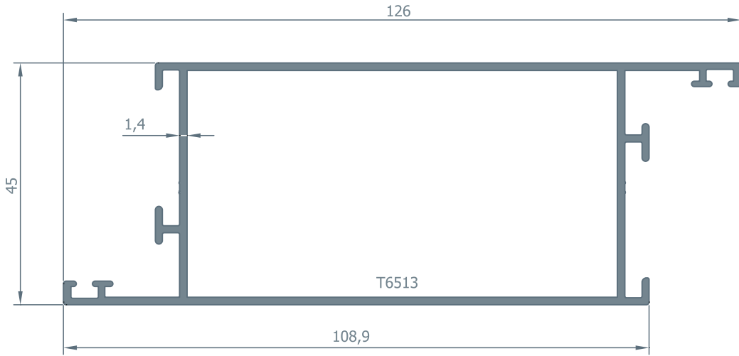
6513 Kapı Kanat Profili 1.295 kg/m
