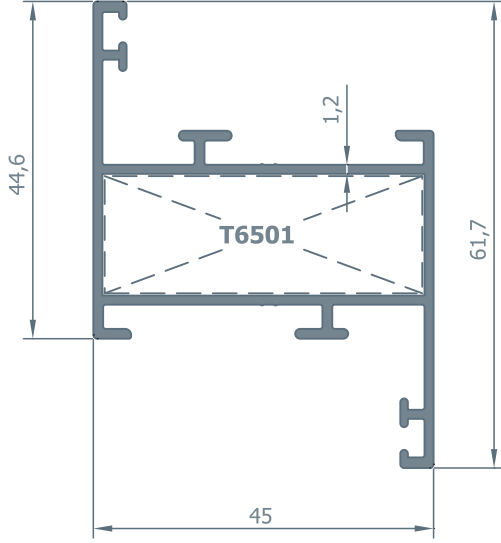
6501 Kanat Profili 0.730 kg/m
