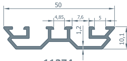
11274 Baskı Profili 0.365 kg/m Jx: 0,13 Jy: 3,15
