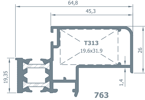
Yalıtımlı Kaset Profili
