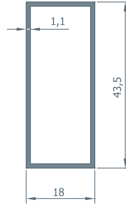
607 0.355 kg/m
