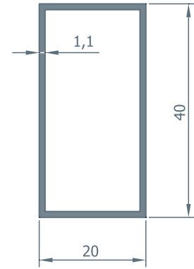
344 0.345 kg/m
