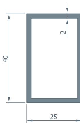
412 0.660 kg/m
