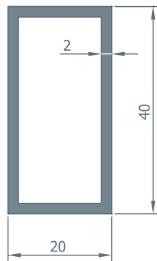
414 0.610 kg/m
