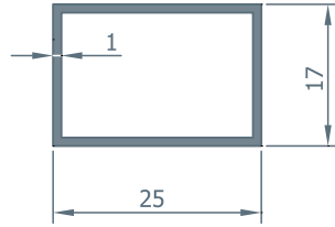
2280 0.218 kg/m
