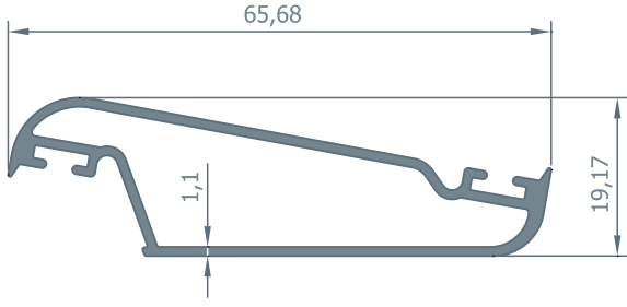
324 Panjur Yaprağı 0.505 kg/m
