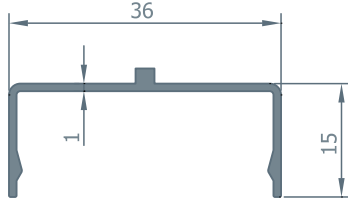
780 Panjur Yan Kapak 0.193 kg/m
