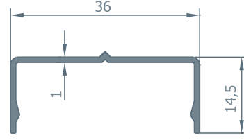
779 Panjur Yan Kapak 0.179 kg/m
