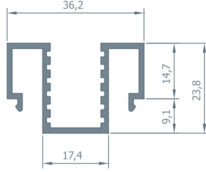
701.98 Panjur Alt Kapak 0.465 kg/m
