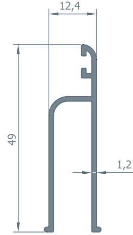
309 Panjur Bitiş Yaprağı 0.331 kg/m
