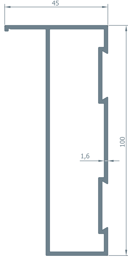
2614 Kasa Profili 1.220 kg/m
