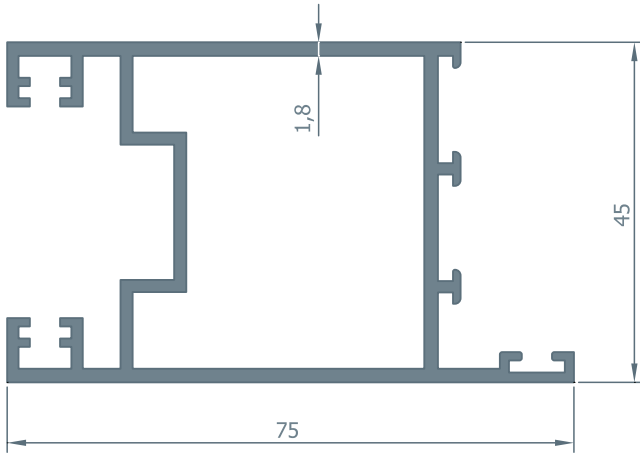
2005 Kanat Profili 1.304 kg/m
